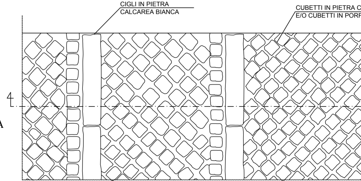
PIANTA
